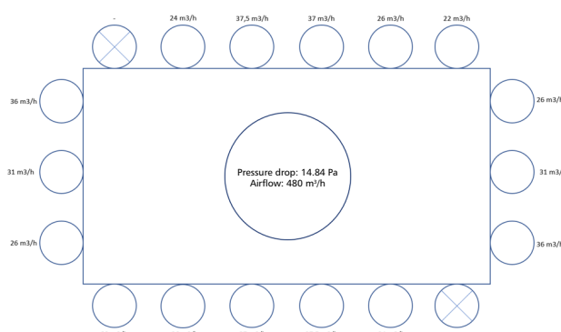
3-5-3-5 (200 mm inlet)
